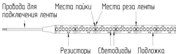
Рисунок 1 – Внешний вид светодиодной ленты Geniled (на примере GL-240SMD2835).
